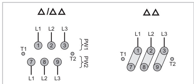
Fig. 37: Possibilités de raccordement du moteur à bobinage partiel
