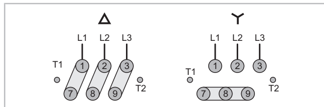
Abb. 40: Direktanlauf-Anschlussmöglichkeiten des Stern-Dreieck-Motors
