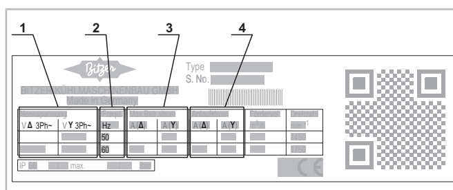
Fig. 18: Compresseur avec moteur à démarrage direct, exemple d'une plaque de désignation
