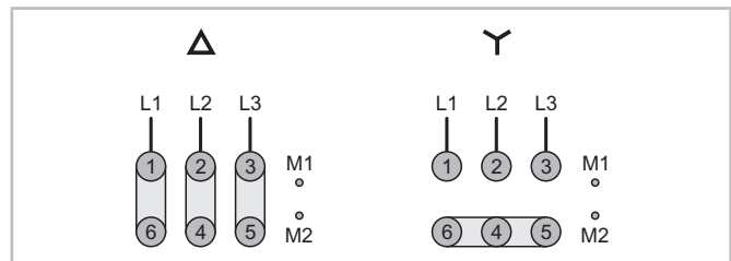
Abb. 26: Anschlussmöglichkeiten des Stern- oder Dreieck-Motors
