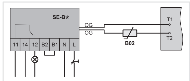
Fig. 42: Circuit de mesure de la température avec SE-B*
