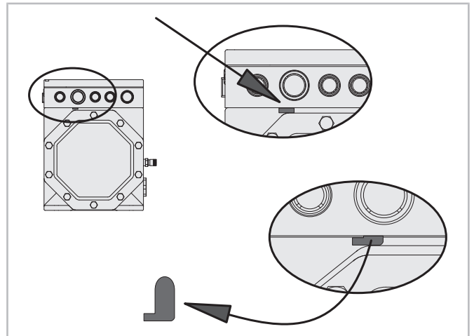
Abb. 47: Beispiel für Ablassstopfen für Kondenswasser am Anschlusskasten
