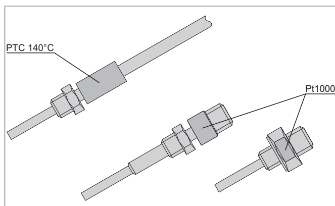
Abb. 13: Position der Typenbezeichnung an Druckgastemperaturfühlern
