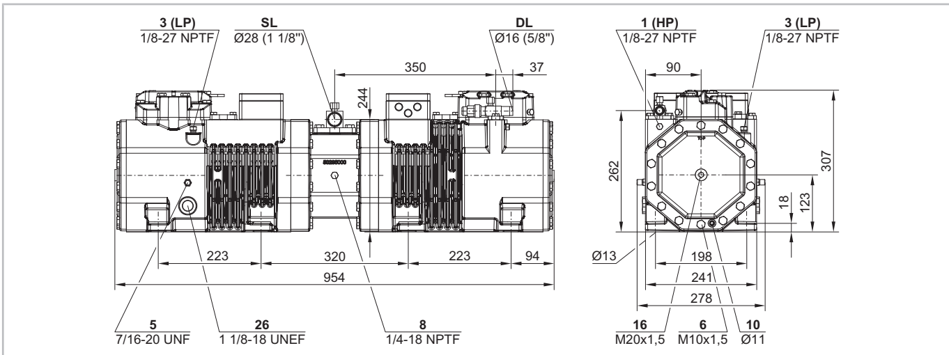
Abb. 15: Maße mit Modulgehäuse siehe Einzelverdichter
