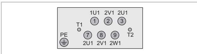
Abb. 36: Stromdurchführungen und innen angeschlossene Motorwicklungen
