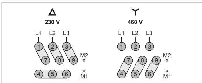
Fig. 35: Possibilités de raccordement pour le démarrage direct du moteur à 9 bornes
