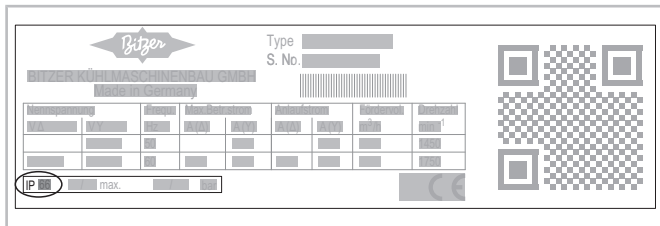
Abb. 41: Links unten auf dem Typenschild befindet sich die Angabe der Schutzart.
