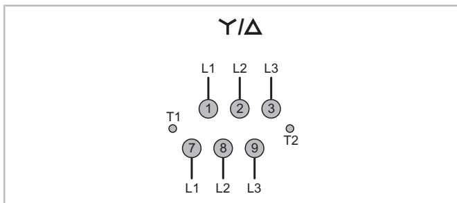
Fig. 39: Raccordement du moteur à étoile-triangle
