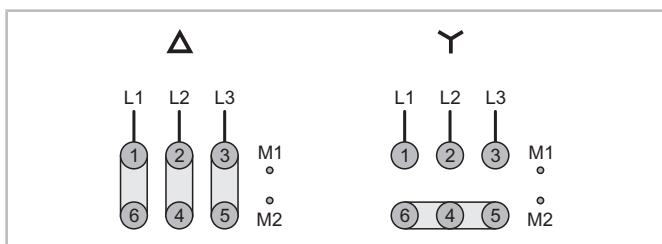
Fig. 26: Possibilités de raccordement du moteur étoile ou triangle
