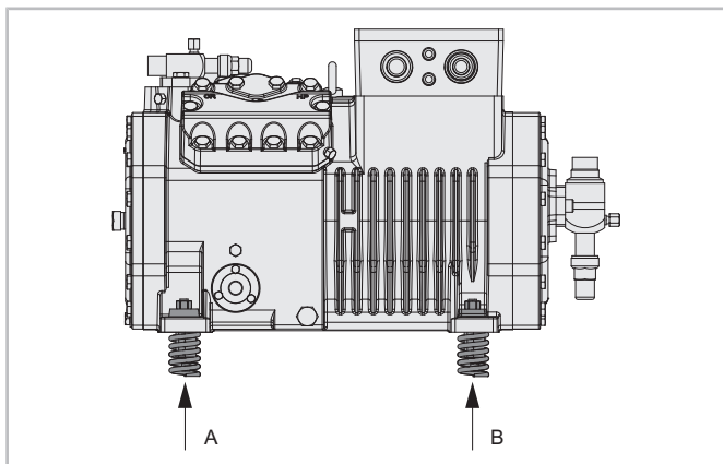
Fig. 12: A: Crankcase side, B: Motor side
