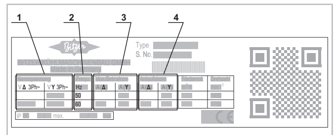
Abb. 18: Verdichter mit Direktanlaufmotor, Beispiel eines Typschilds
