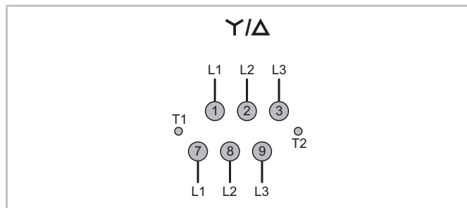
Abb. 39: Anschluss des Stern-Dreieck-Motors
