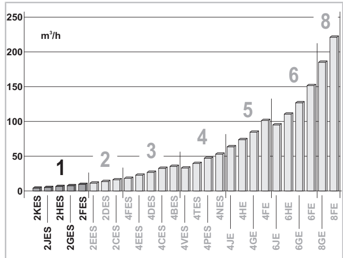
Abb. 7: Verdichterübersicht: Fördervolumina bei 50 Hz, die verfügbaren Verdichtertypen sind dunkelgrau dargestellt.
