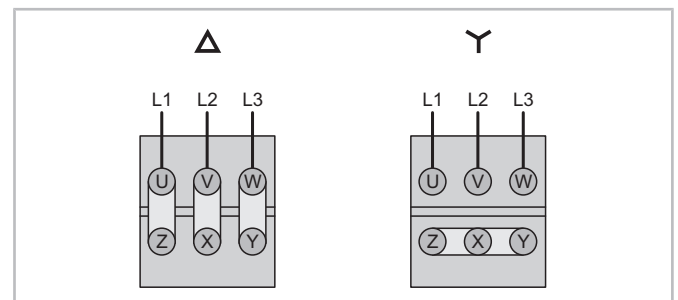
Abb. 22: Anschlussmöglichkeiten des Stern- oder Dreieck-Motors
