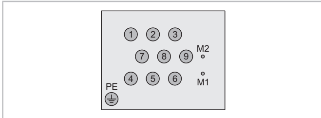
Fig. 33: Passage de courant du moteur à 9 bornes
