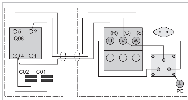
Fig. 23: À gauche : relais de démarrage, à droite : boîte de raccordement avec passages de courant gris clair, câblage dans l'état à la livraison vers le bornier, gris plus foncé. Les enroulements du moteur raccordés à l'intérieur y sont indiqués.
