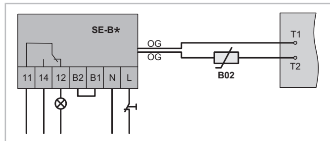
Abb. 42: Temperaturmesskreis mit SE-B*
