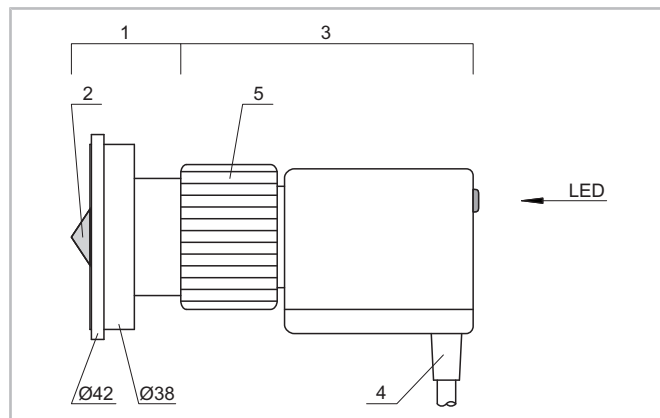
Abb. 5: Aufbau des OLC-D1
