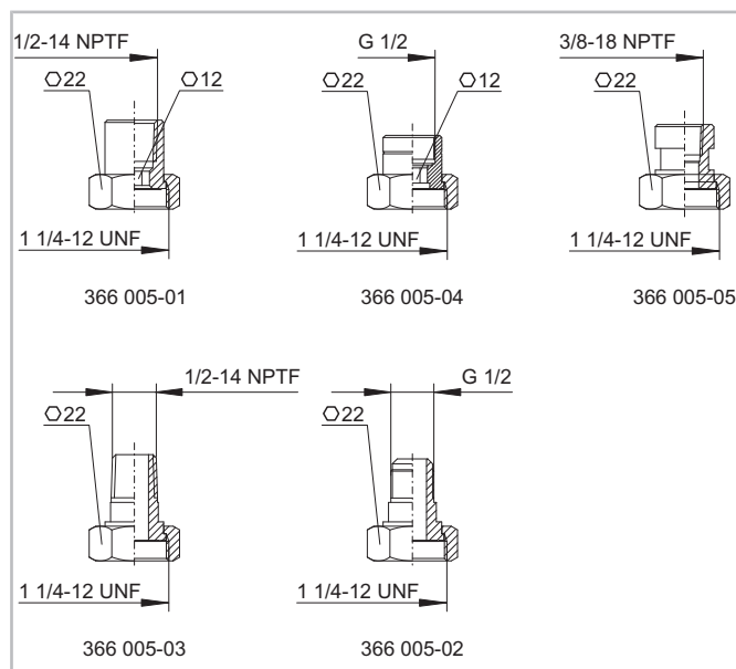
Abb. 4: Adapter für das Druckentlastungsventil
